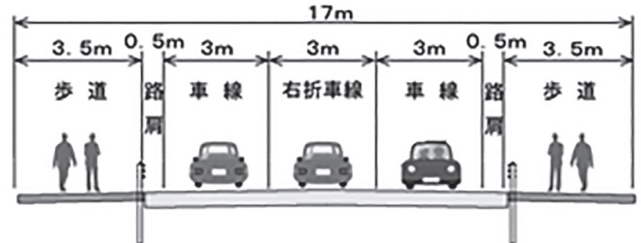
計画平面図 (小渕江南線・浅井犬山線)
