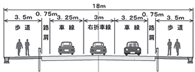
標準横断図 (小渕江南線 交差点部)
