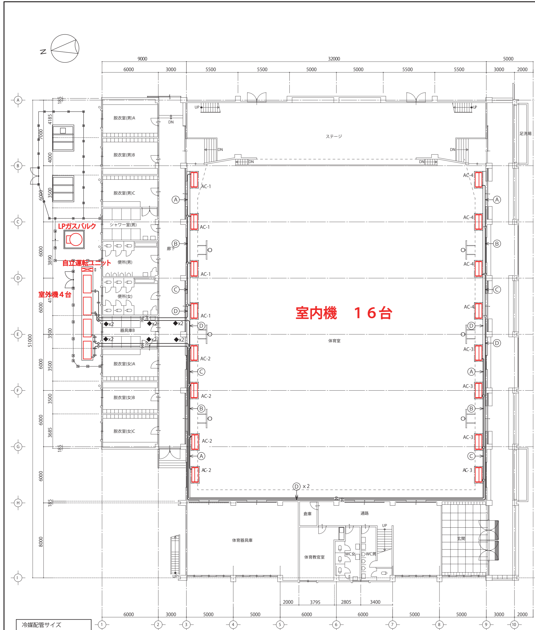
1階平面図 1/200
