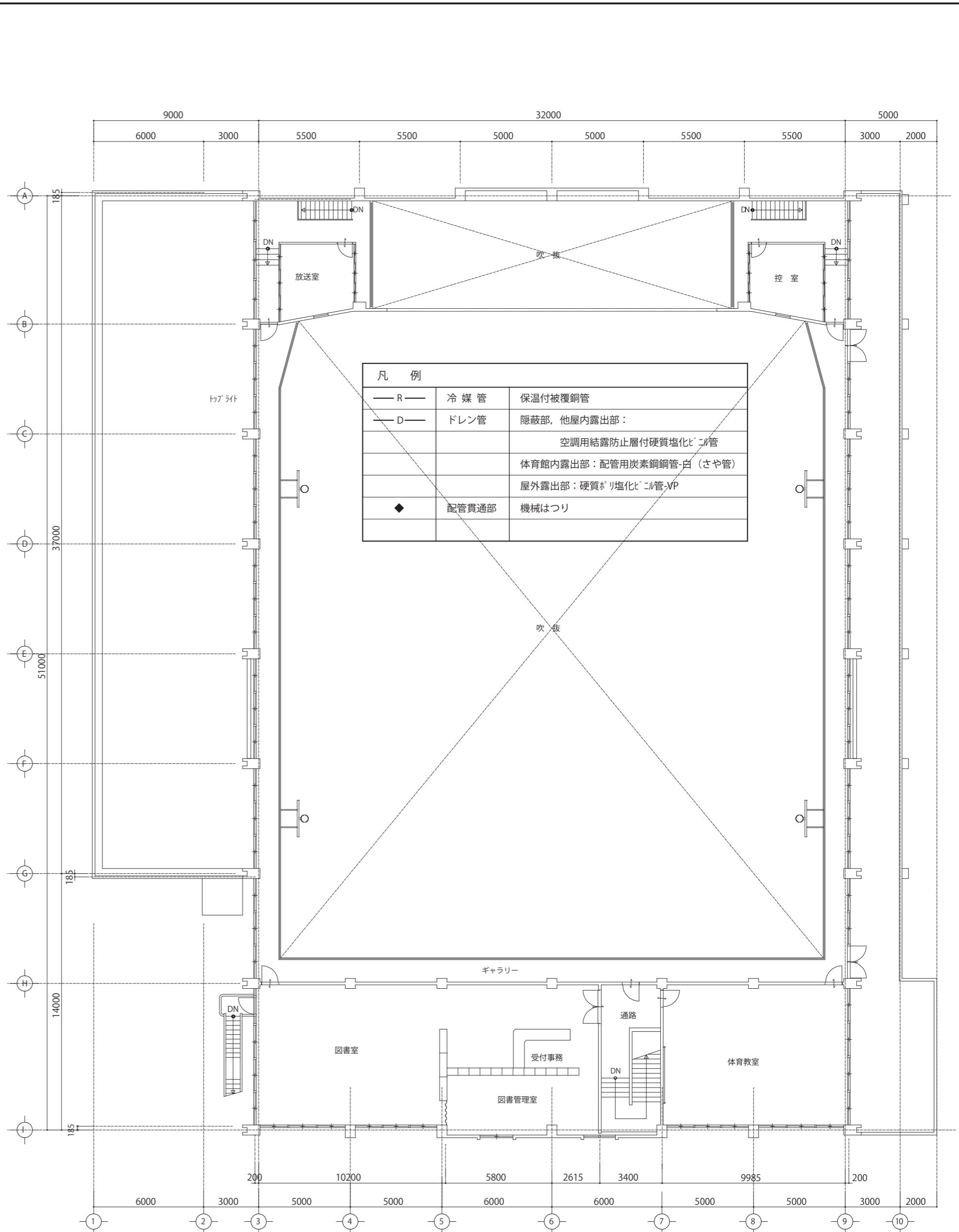
2階平面図 1/200
